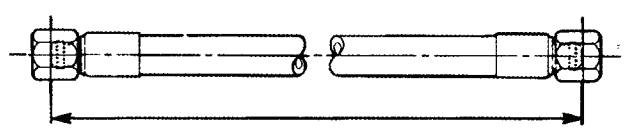
Länge über Dichtkegel Overall length over female swivel
